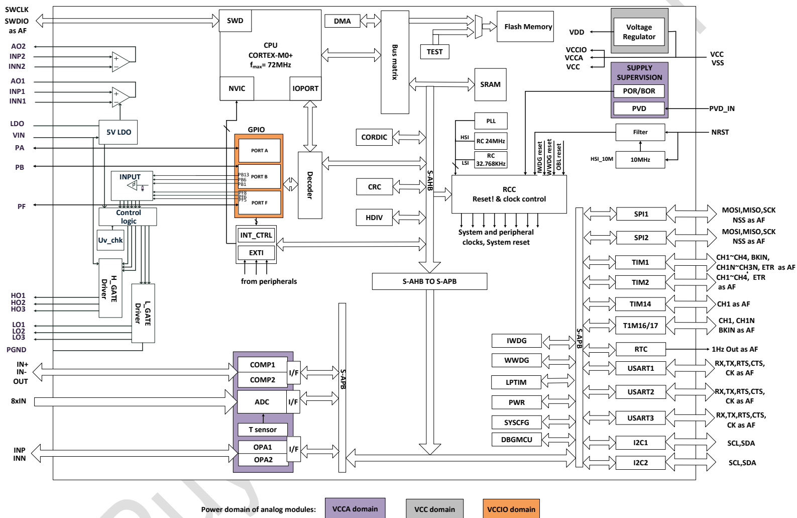
图 1-1 功能模块
