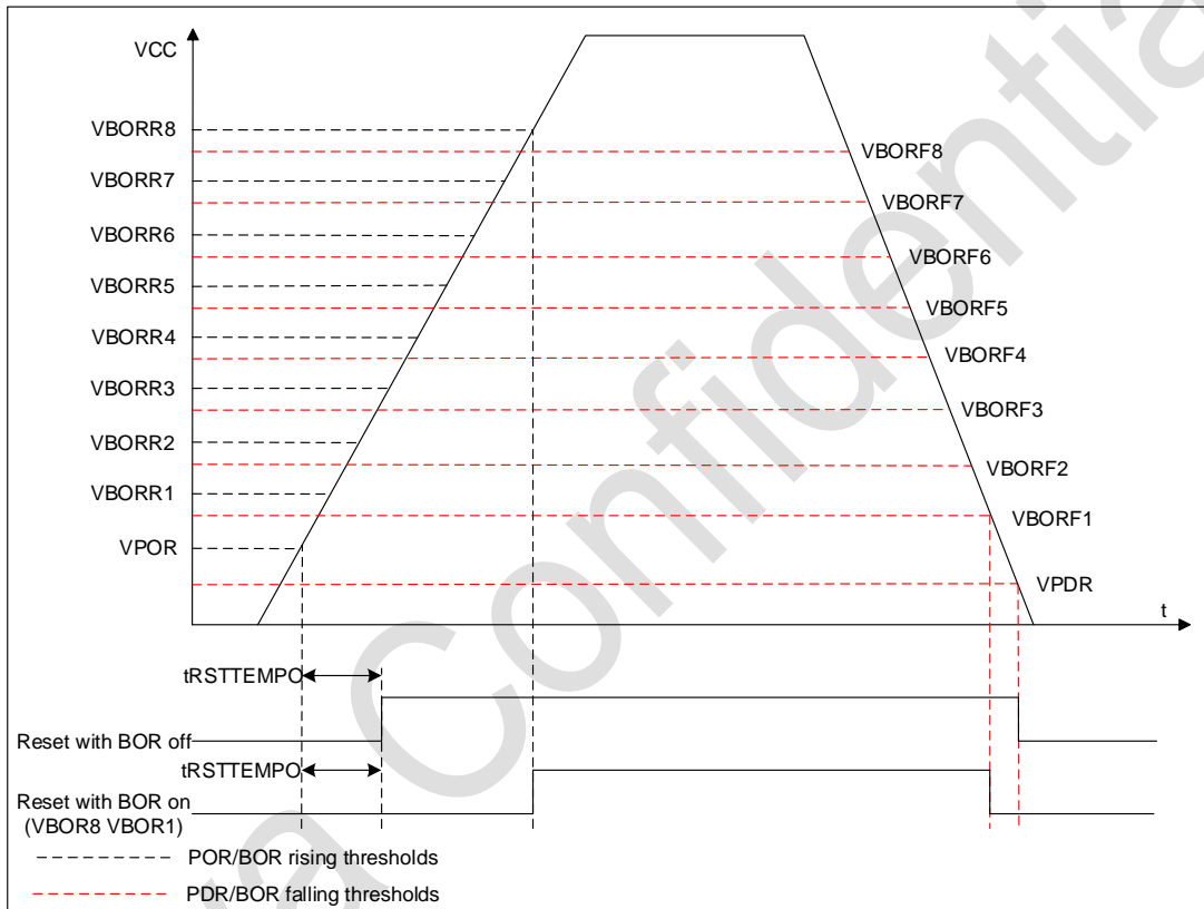
图 2-3 POR/PDR/BOR 阈值
